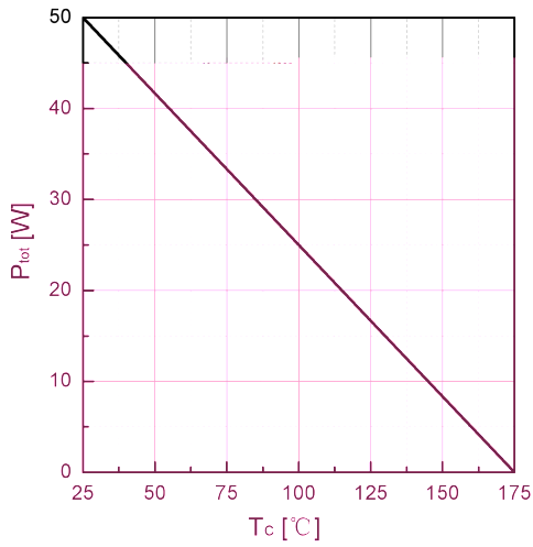
T_c
